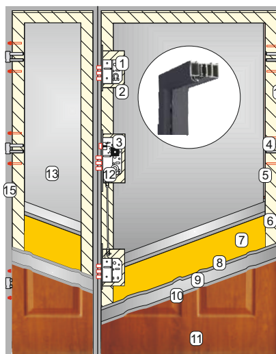
Dostawka nie otwierana
