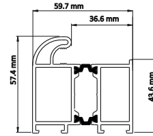
Profil ościeżnicy KMT ENERGY 60
