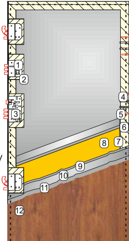
KMT Plus 75 max
