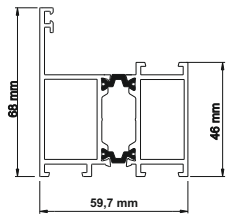
Profil progu ENERGY 60
