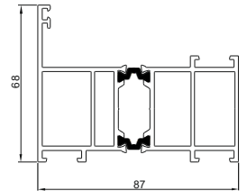
Profil progu ENERGY 90
