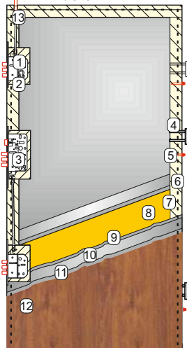
KMT Plus 54 kl.2
